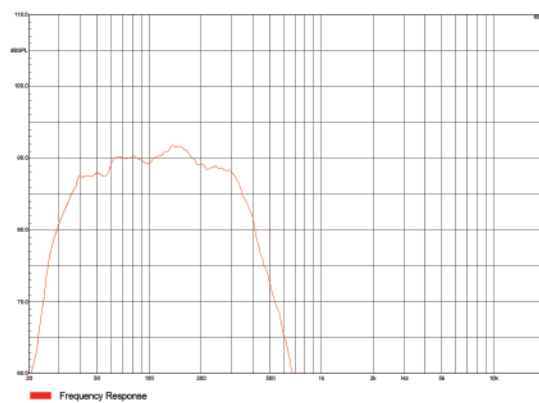
① Artist TW8频响曲线图
